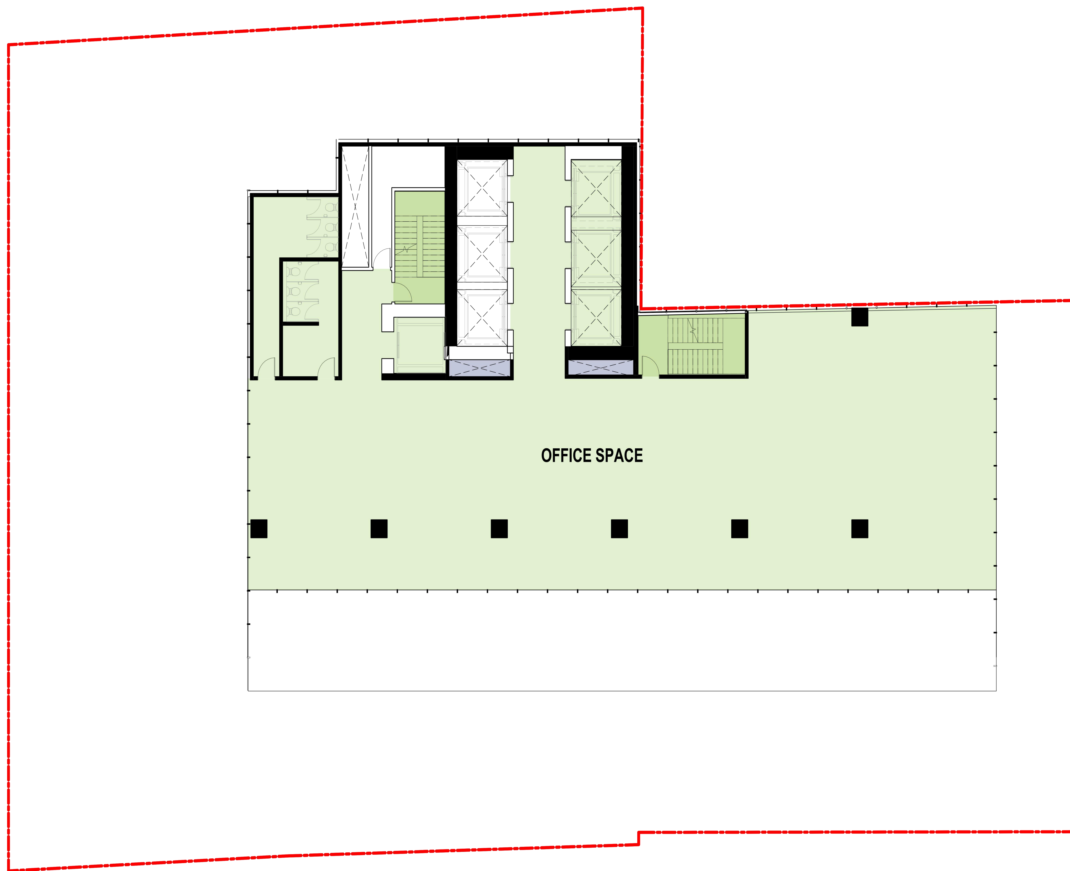
30- FFL-OSD Level 1:100
